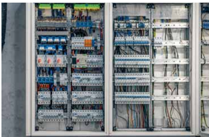
Fixation de tableaux électriques industriels
